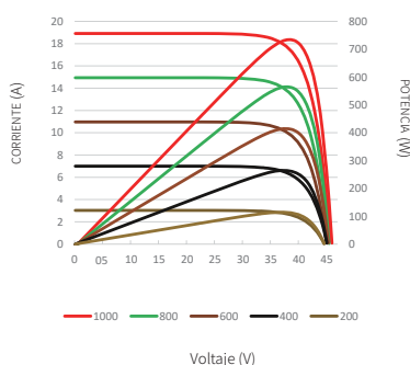
Curvas de corriente-voltaje y potencia-voltaje (720W)
